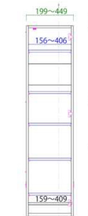
幅調整キャビネット L 幅調整キャビネット R
