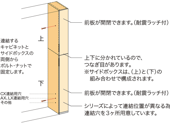
サイドボックス上下(右)を設置した図
